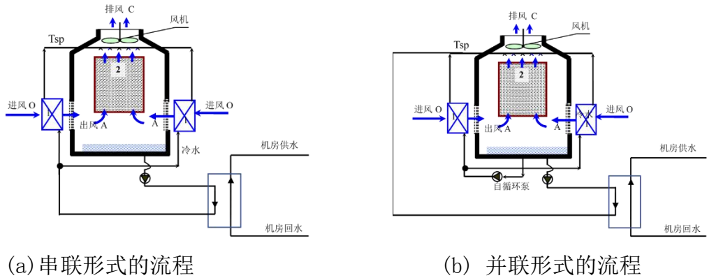
图 9. 利用间接蒸发冷水机流程制备冷水排走机房热量
