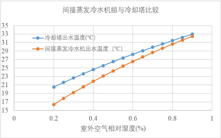
图 6. 间接蒸发冷水机组与常规冷却塔的比较（室外干球温度为 34℃，填料塔 NTU=3）
