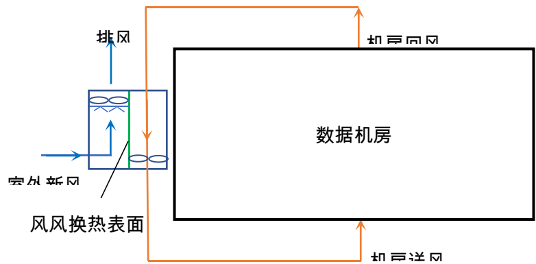
图 1. 新风直接蒸发冷却方式，冷却机房回风
