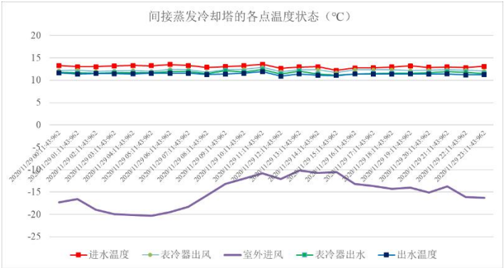
图 14. 2020 年 11 月底典型日的间接蒸发冷却塔运行状态
