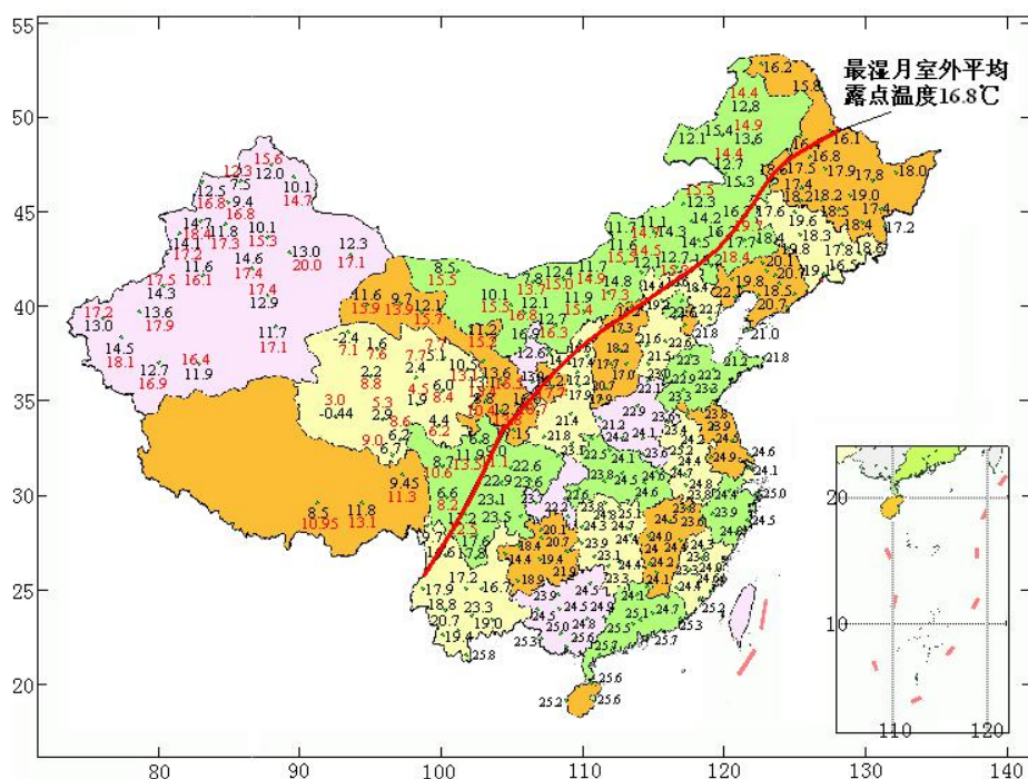
图 5. 我国西北各地最湿月室外平均露点温度和间接蒸发冷水机组出水温度
