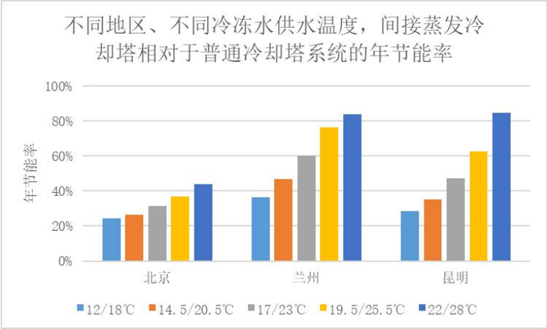
图 18. 间接蒸发冷却与机械制冷结合的方式与普通水冷系统相比的节能效果
