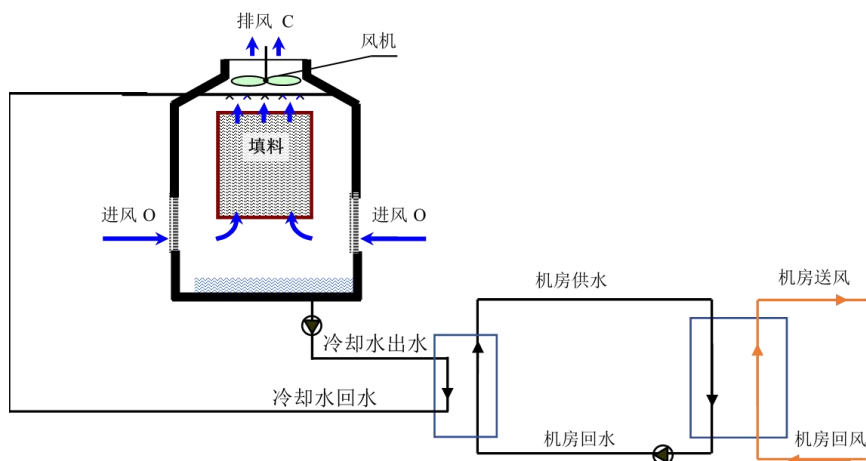
图 2. 利用冷却塔制备冷水实现机房排热的系统
