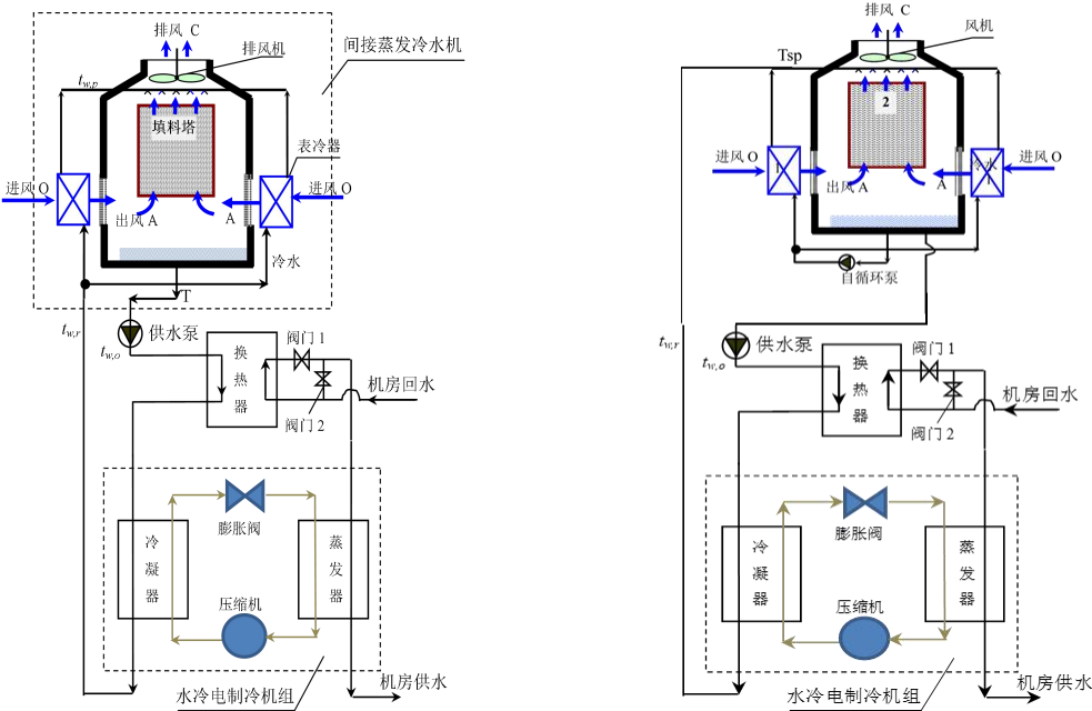
(a) 串联式间接蒸发冷水机组与电制冷结合 (b) 并联式间接蒸发冷水机组与电制冷结合
