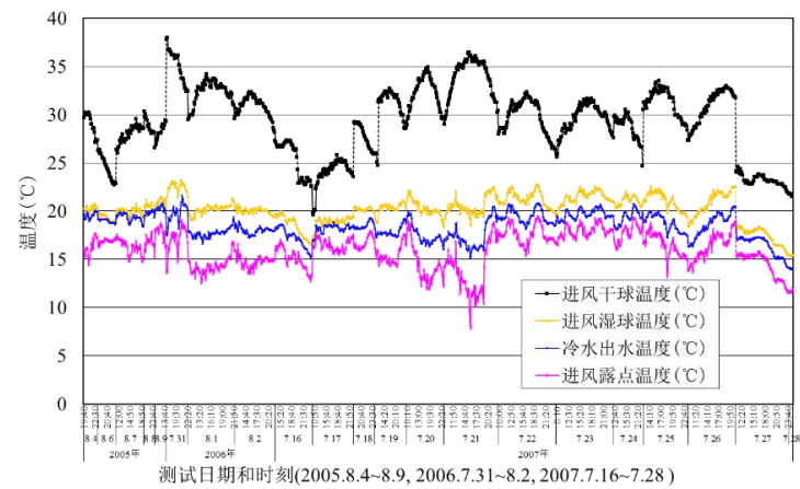
图 4. 间接蒸发冷水机组实测出水温度
