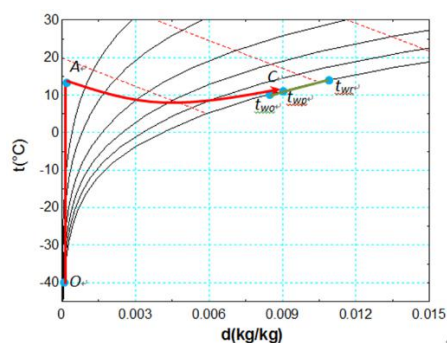
图 10. 间接蒸发冷却塔在-40℃下的排热过程举例
