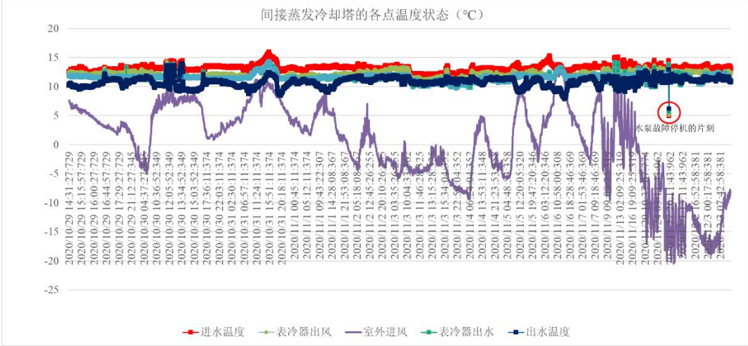
图 13. 2020. 11~2020. 12 间接蒸发冷却塔的运行状况
