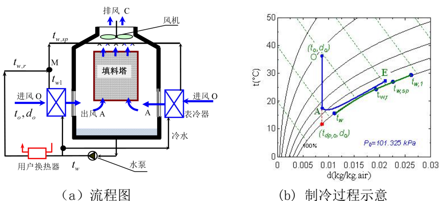
图 3 间接蒸发冷却制备冷水的原理
